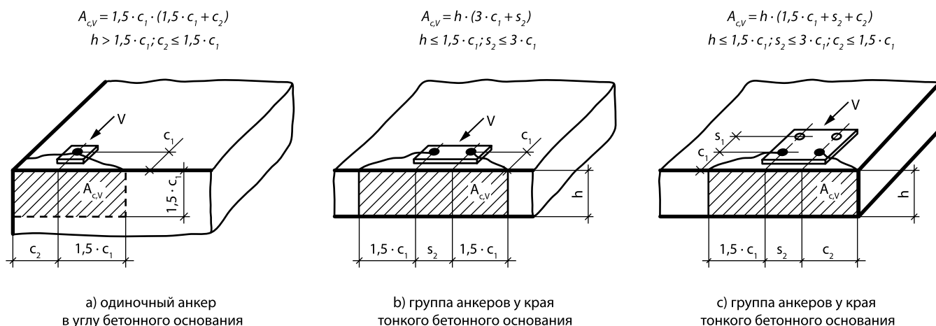
Рисунок 1.7 Фактическая площадь основания условной призмы выкалывания для одиночных анкеров и анкерных групп при сдвиге
