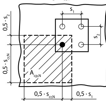
а) анкер в группе вдали от края
