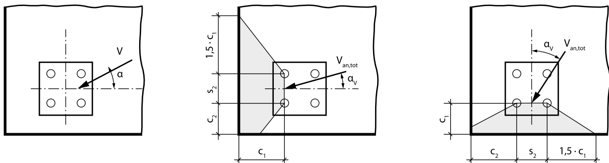
Рисунок 1.9 Расчетные схемы при проверке откалывания края основания вблизи угла
