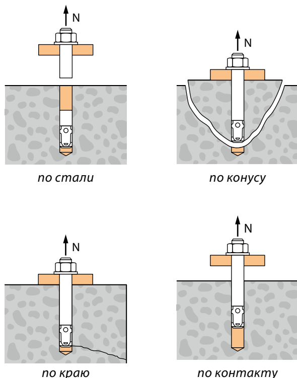
Рисунок 1.1 Виды разрушений при вырывающем усилии
