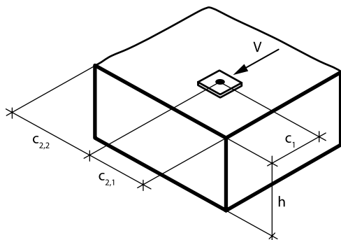
Рисунок 1.10 Обозначение параметров взаимного расположения одиночного анкера
