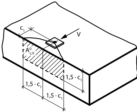
Рисунок 1.8 Площадь A_{c,V}^0 основания условной призмы выкалывания при сдвиге для одиночного анкера, расположенного на значительном удалении от угла основания и соседнего анкера
