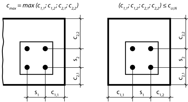
Рисунок 1.5 Схема расположения анкеров в стесненных условиях
