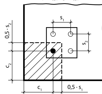
в) анкер в группе из четырех анкеров в углу бетонного основания
