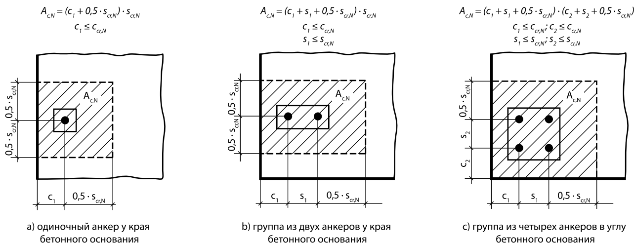
Рисунок 1.3 Фактическая площадь основания условной призмы выкалывания для одиночного анкера и анкерных групп при действии растягивающих усилий
