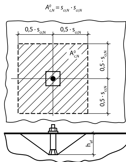
Рисунок 1.4 Площадь основания условной призмы выкалывания при растяжении для одиночного анкера, расположенного на значительном удалении от края основания и соседнего анкера
