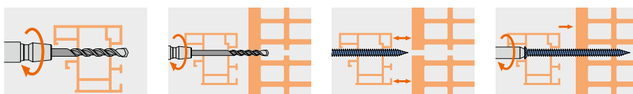
MRS Стеновой шуруп, головка 11,5 мм
