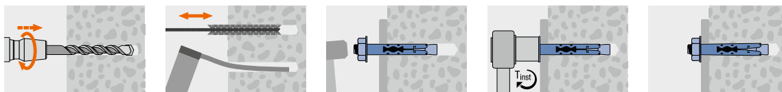
MNA-S Анкер-гильза (болт, оцинкованная сталь)
